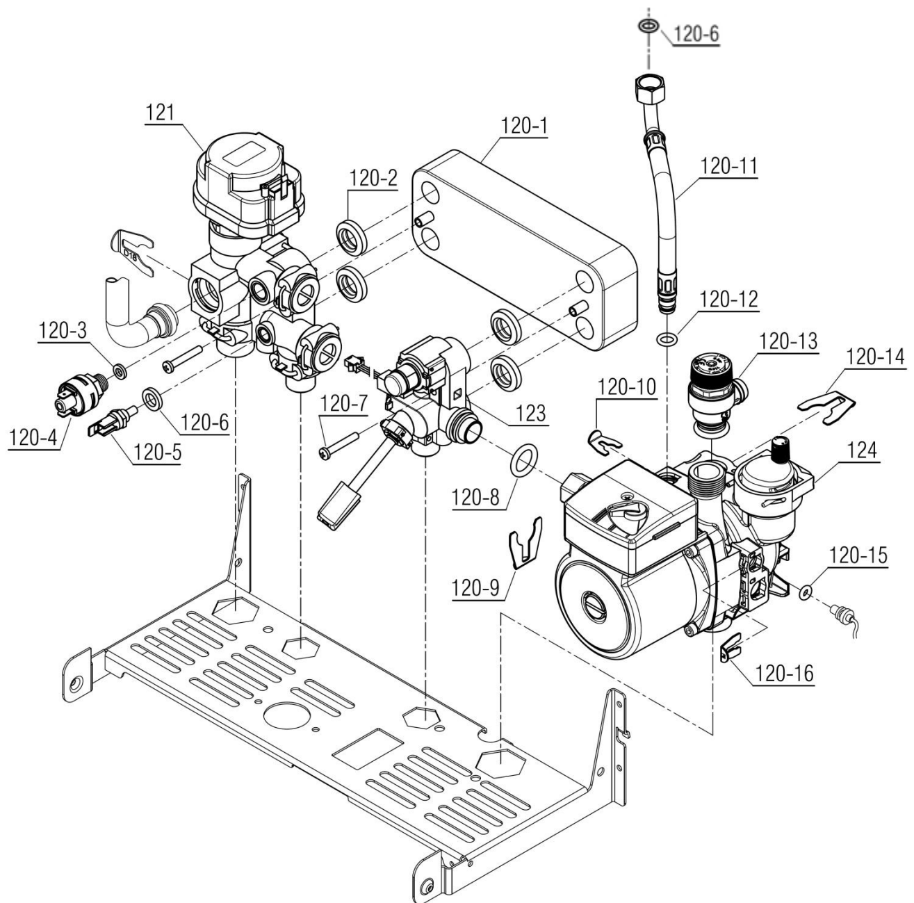
مجموعه مدار هیدرولیک Irturpan 26S Digital 120
